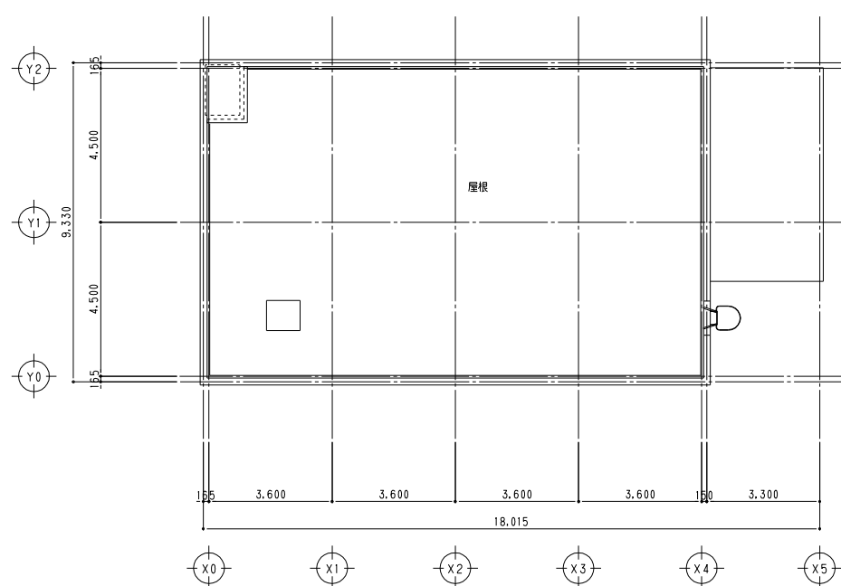
A1:1/100 A3:1/200
