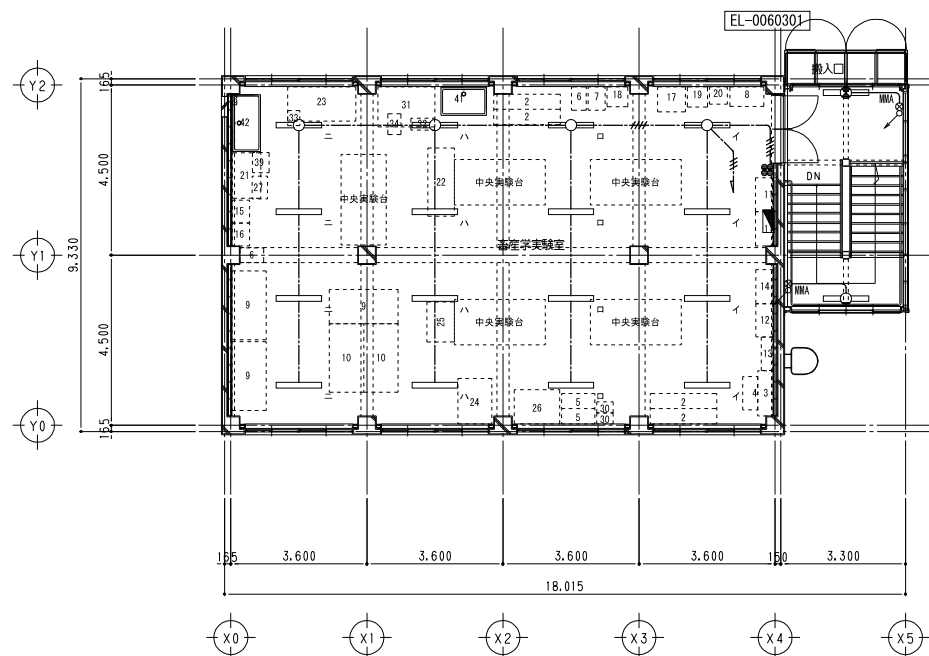
A1:1/100 A3:1/200
